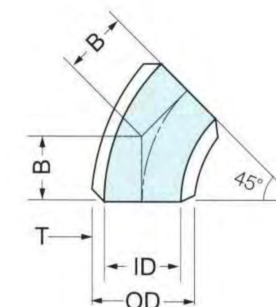
45° Elbow
