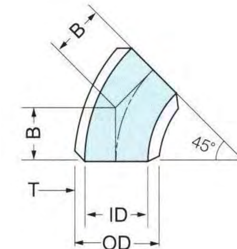
45° Elbow
